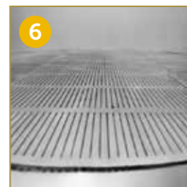
PIASTRA FILTRANTE ESTRAIBILE CON TAGLI TRAPEZOIDALI (0,75-1,2 MM.)
